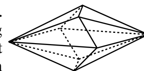
Fig. 3. Skalenoeedrisk calcitkrystal.
